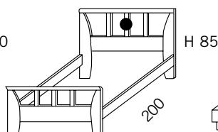
Letto bastoncini Wooden stick bed
